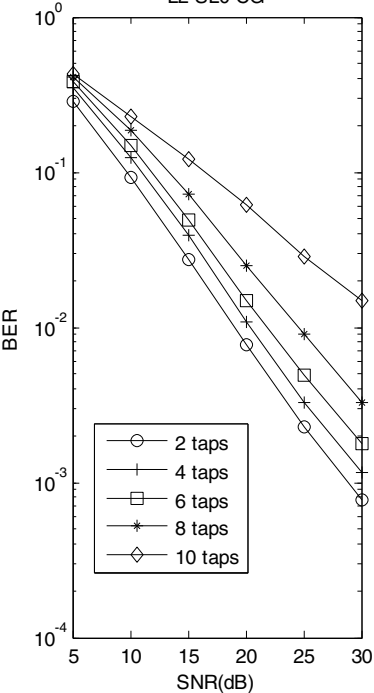
L2-SL0-CG
