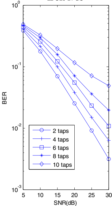
L2-SL0-BFGS
