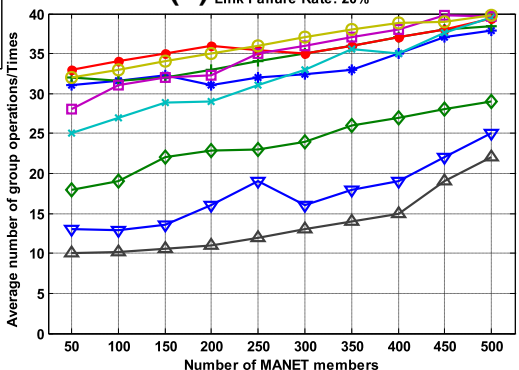
(d) Link Failure Rate: 20%
