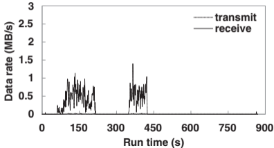
Map node
