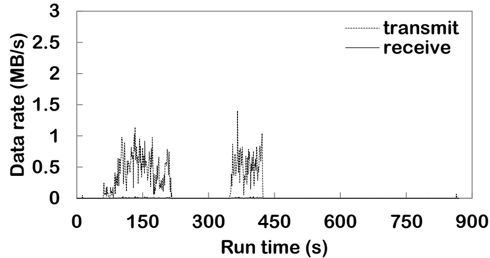
Map node
